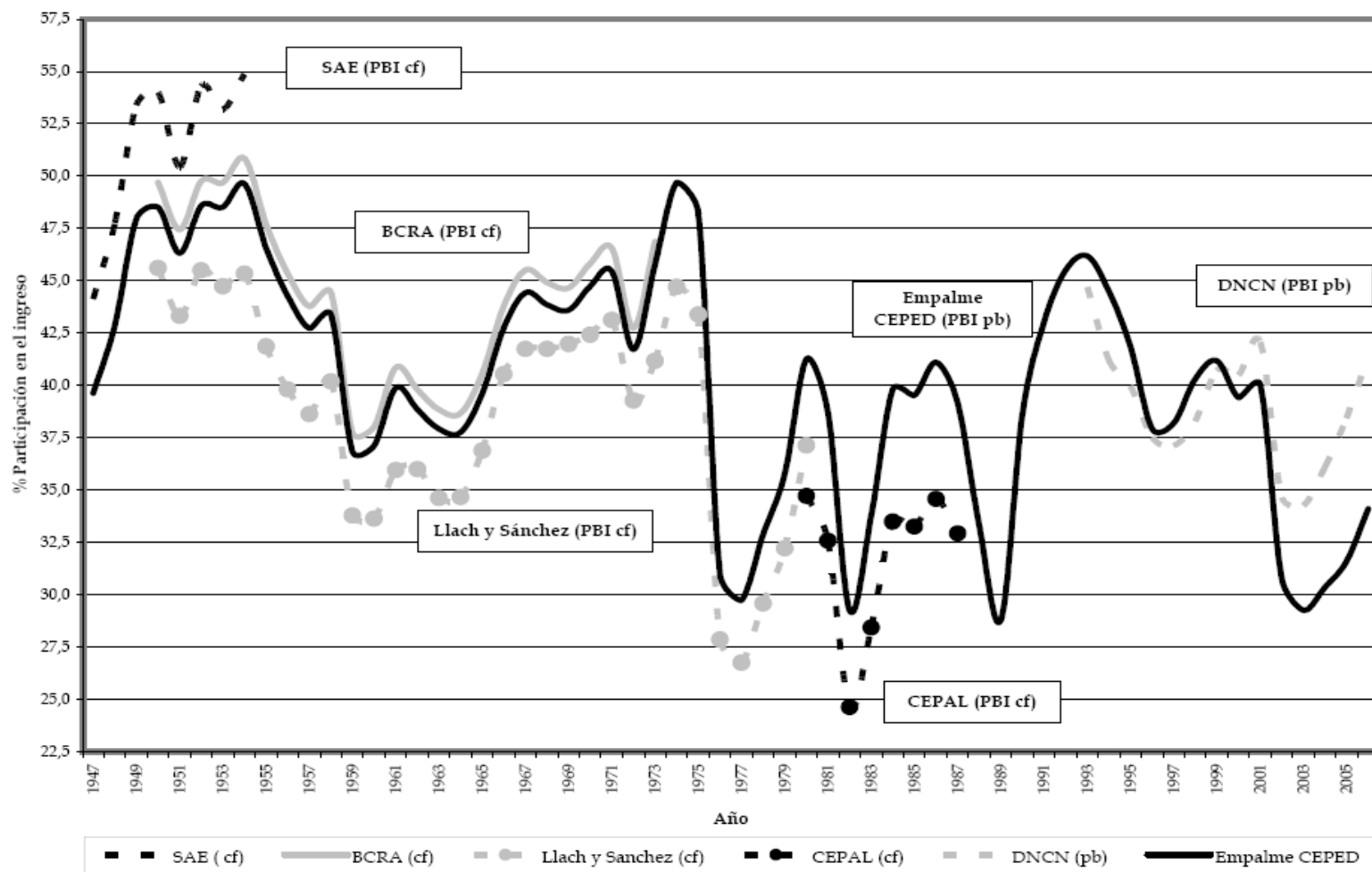
GRÁFICO 1. Participación salarial en el PBI a costo de factores o precios básicos. Series seleccionadas y Empalme CEPED. En porcentaje. 1947 - 2006.
